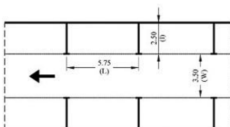
Figura 6.3 Parcarea pentru autoturisme
