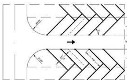
Figura 6.2 Parcarea la 45°, 60° sau 75° cu cale de acces cu sens unic de circulație
