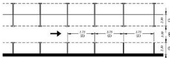
Figura 5.7 Parcarea longitudinală cu cale de circulație cu sens unic sau dublu
