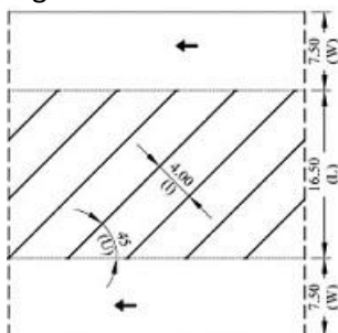
Figura 6.8 Parcare autovehiculelor articulate la 45°
