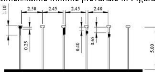
Figura 5.2 Parcare la 90° alăturată unor elemente de construcție poziționate la o distanță cuprinsă între 0
