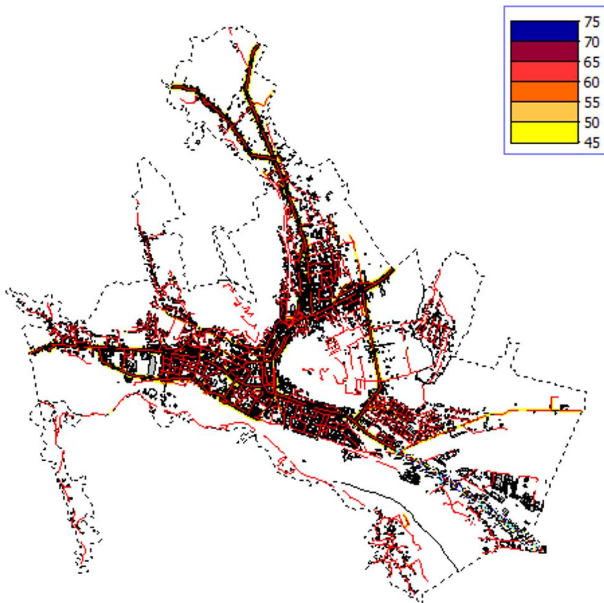
Figura 2. Harta depășiri valori de prag zgomot trafic rutier pentru parametrul Lnoapte
