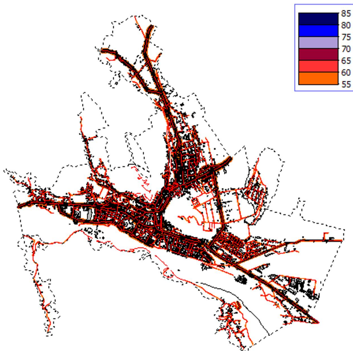
Figura 1. Harta depășiri valori de prag zgomot trafic rutier pentru parametrul Lzsn
