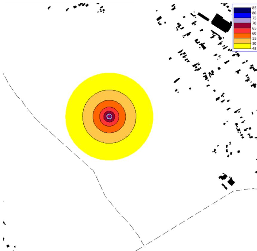
Figura 9. Harta depășiri valori de prag zgomot produs de Depozit Deșeuri Piatra Neamț pentru parametrul L zsn
