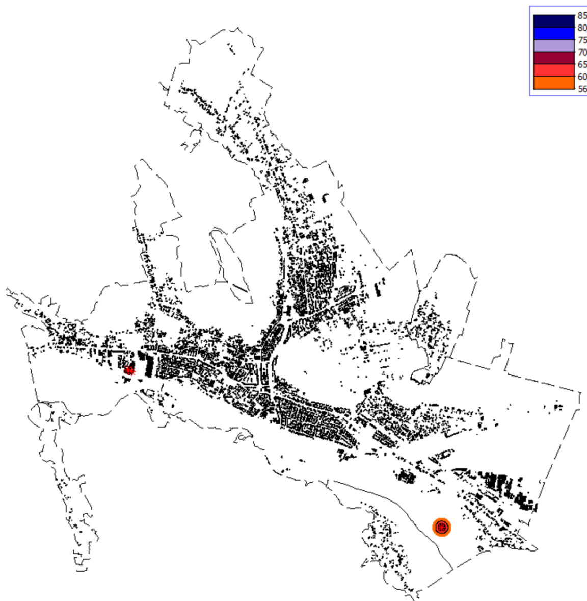
Figura 5. Harta depășiri valori de prag zgomot industrie pentru parametrul Lzsn
