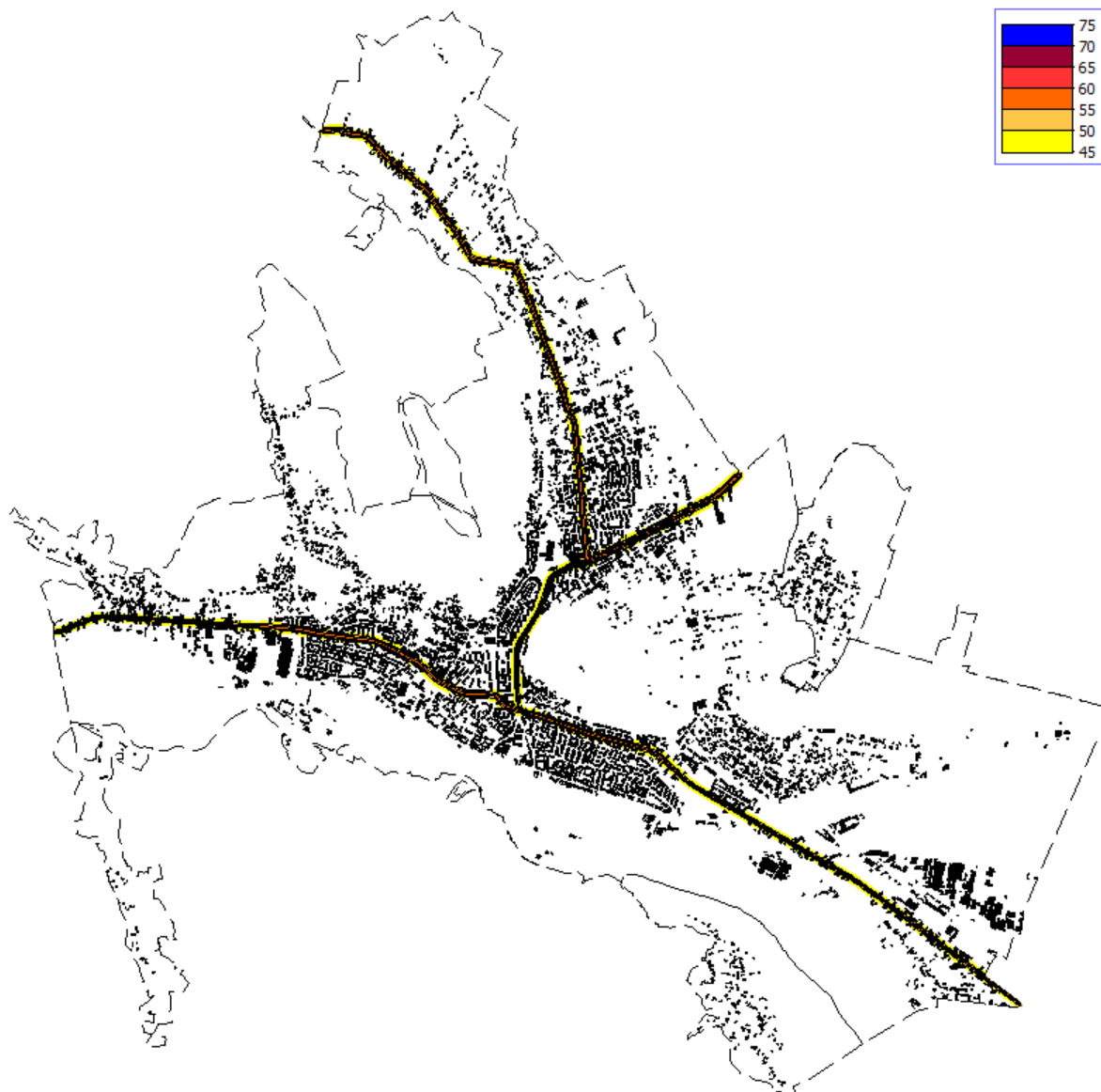
Figura 4. Harta depășiri valori de prag zgomot trafic rutier – drumuri principale pentru parametrul Lnoapte
