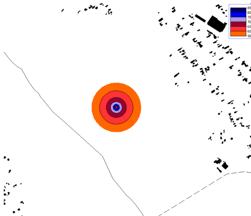
Figura 9. Harta depășiri valori de prag zgomot produs de Depozit Deșeuri Piatra Neamț pentru parametrul L zsn
