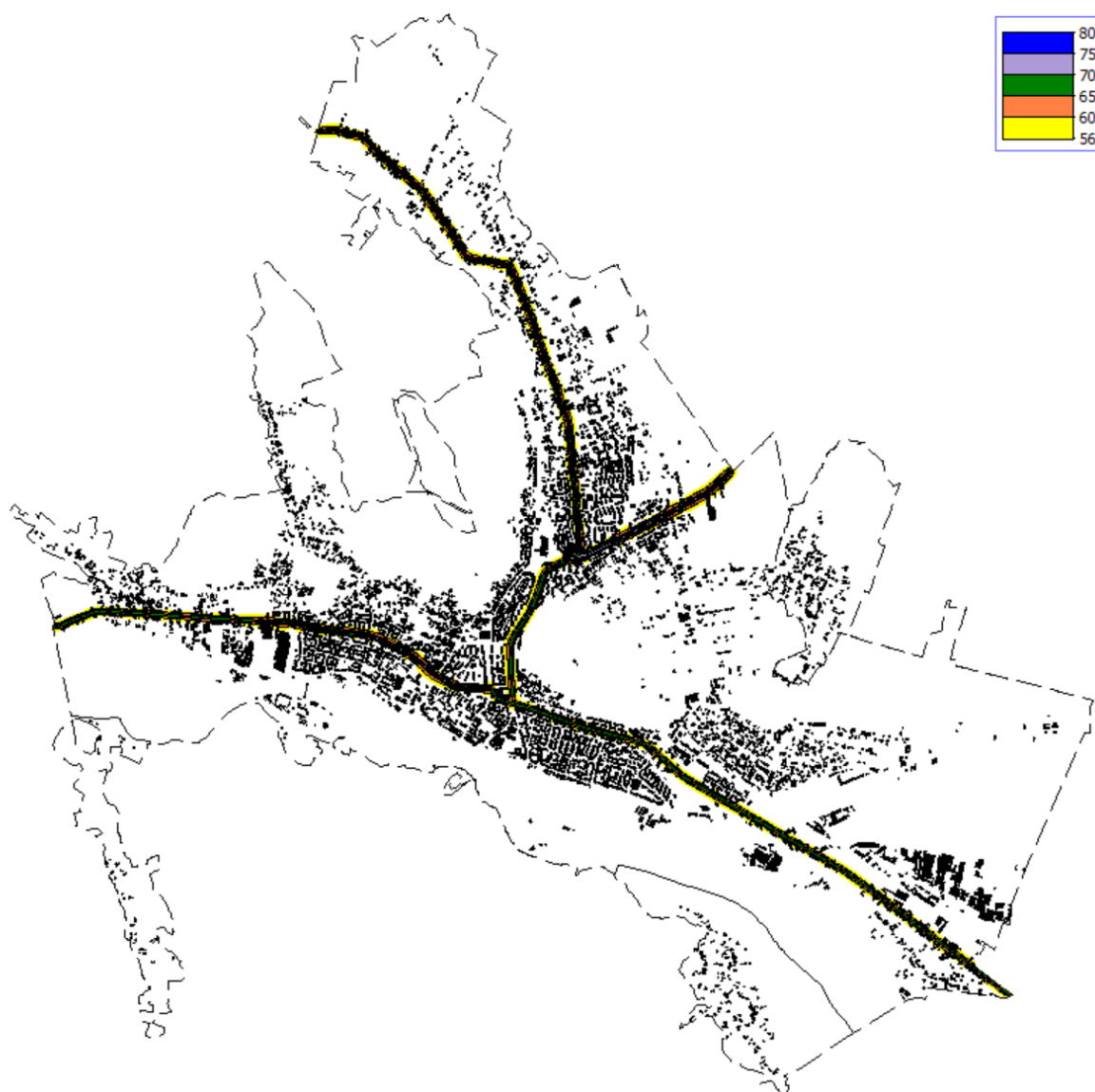
Figura 3. Harta depășiri valori de prag zgomot trafic rutier – drumuri principale pentru parametrul Lzsn
