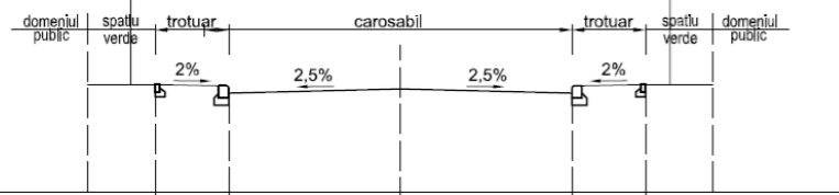
PROFIL TRANSVERSAL amenajare acces str. Mihai Stamatîn
