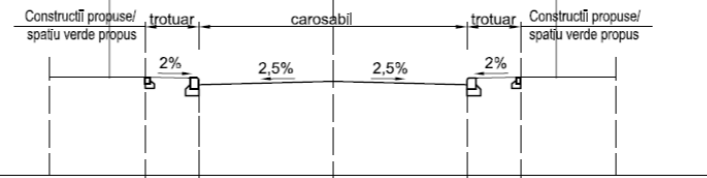
PROFIL TRANSVERSAL amenajare acces str. Constantin Brancoveanu
