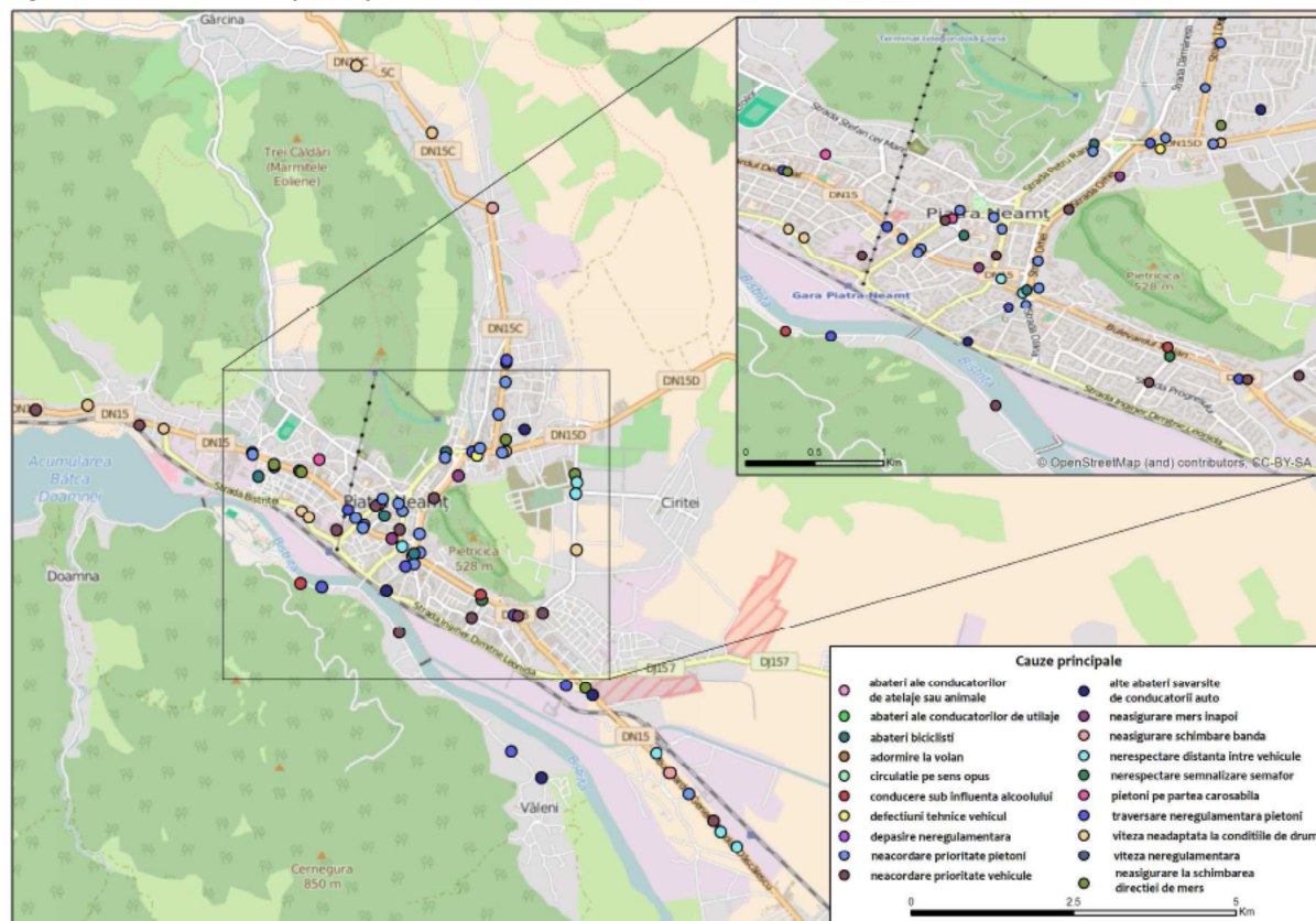
Figura nr. 37: Cauzele principale ale accidentelor (anul 2015)
